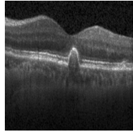
variation_1.png
