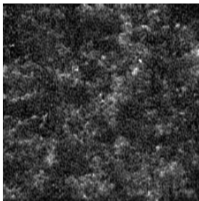
vae_sample_0.png
