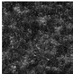
vae_sample_1.png
