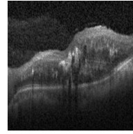
variation_3.png
