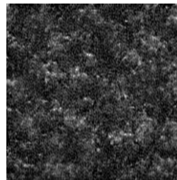
vae_sample_2.png
