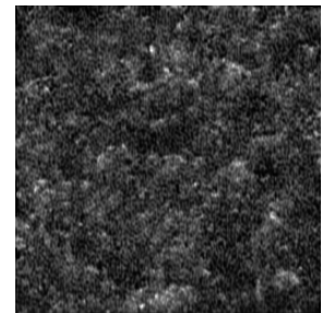
vae_sample_3.png
